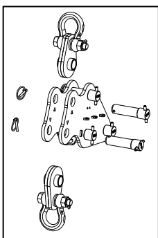
Fixation des dispositifs de centrage au PTILT arrière
