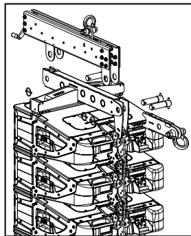
Liaison VBUMP + XBOW pour incl. positive
