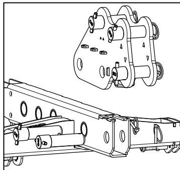
Montage des PTILT sur XBOW
