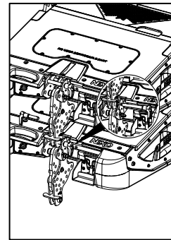
Verrouillage arrière sur M28
