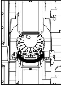
Préréglage d'angle sur M46&B112 et passage en mode "Operation"
