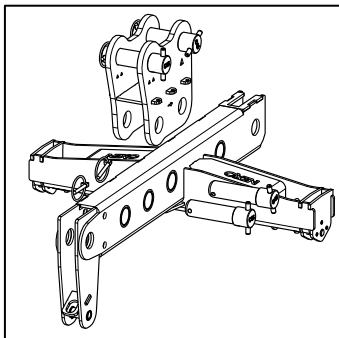
Fixation du MLINK au XBOW ou MBEAM
