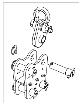
Dispositif de centrage
