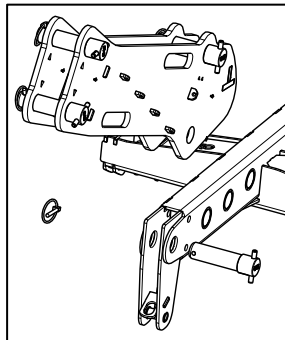
Montage de la KBEAM arrière sur le XBOW ou la MBEAM
