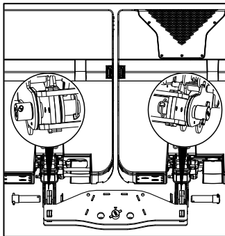
Couplage de 2 BTBUMPER avec BCOUP2
