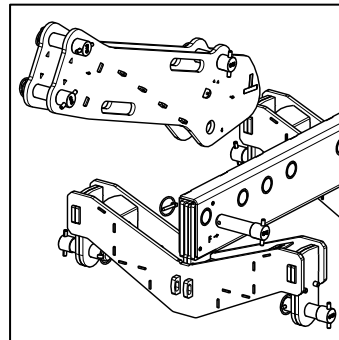
Montage de la KBEAM arrière sur le XBOW ou la MBEAM
