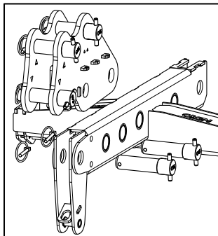
Montage des PTILT sur XBOW
