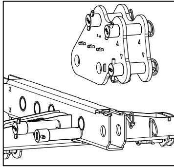
Fixation des PTILT au XBOW
