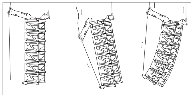
Application de la compression et réglage de l'angle du bumper
