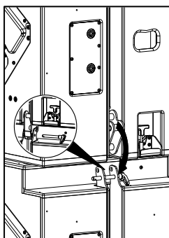
Verrouillage arrière sur S118
