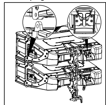
Verrouillage avant sur M28
