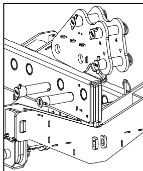
Mise en place du PTILT avant sur la XBOW ou la MBEAM
