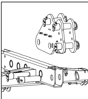
Mise en place du PTILT avant sur la XBOW ou la MBEAM
