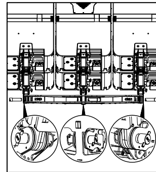
Couplage de 3x BTBUMPER avec BCOUP3
