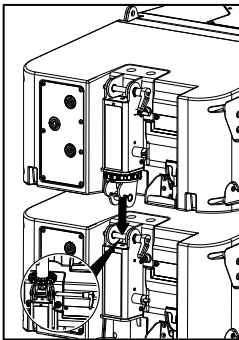
Verrouillage arrière sur B112 et M46
