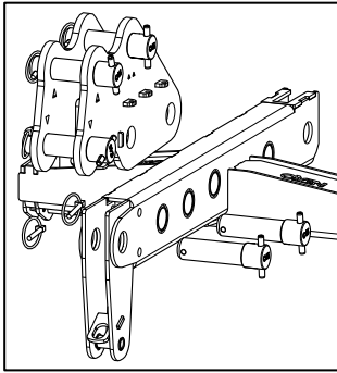
Fixation des PTILT au XBOW
