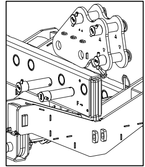
Fixation des PTILT au MBEAM
