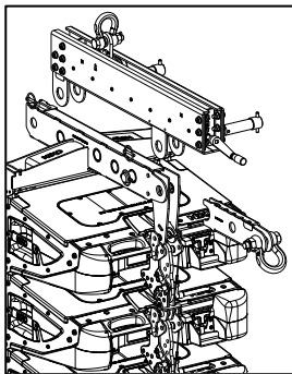
Liaison VBUMP + XBOW pour incl. négative
