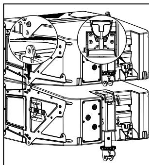
Verrouillage avant sur B112 et M46
